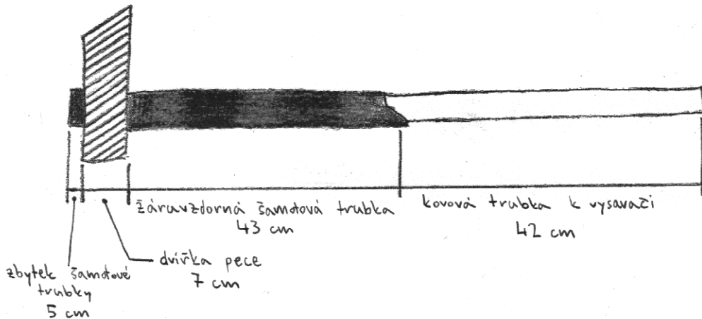
POHLED ZBOKU
